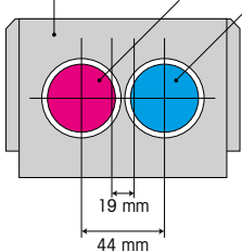
Druckring für 2x Farb-/Rakeltopf Ø 30 mm
