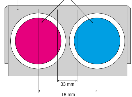
Druckring für 2x Farb-/Rakeltopf Ø 90 mm
